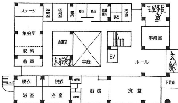
1 階平面図
